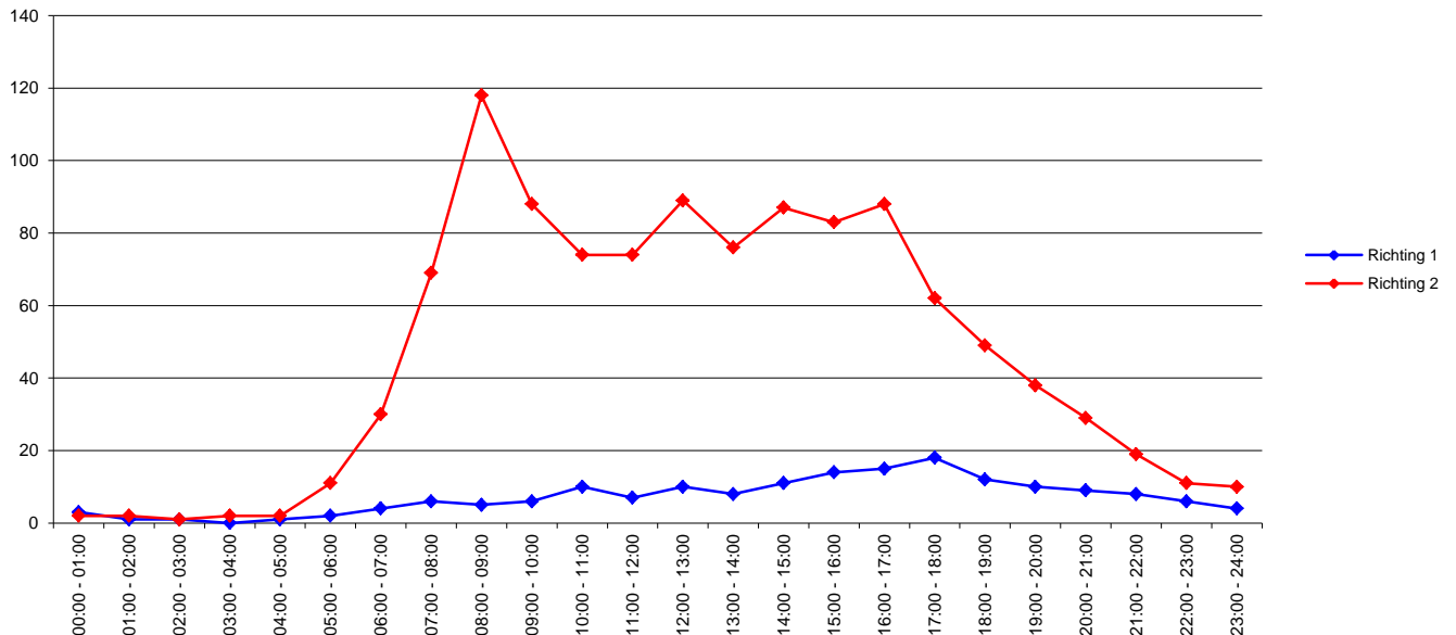
Uurverloop werkdag
