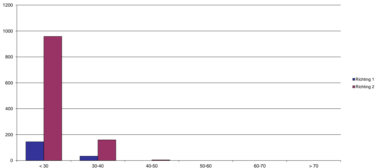
Snelheden werkdag
