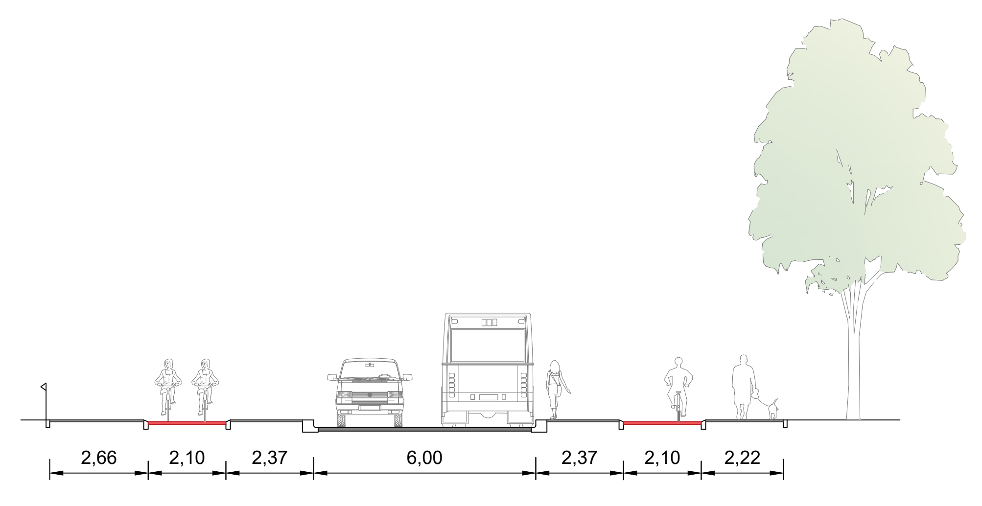
DOORSNEDE B-B schaal 1:100
