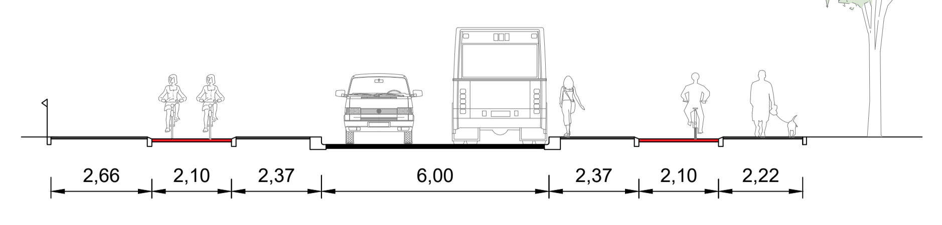
DOORSNEDE B-B schaal 1:100
