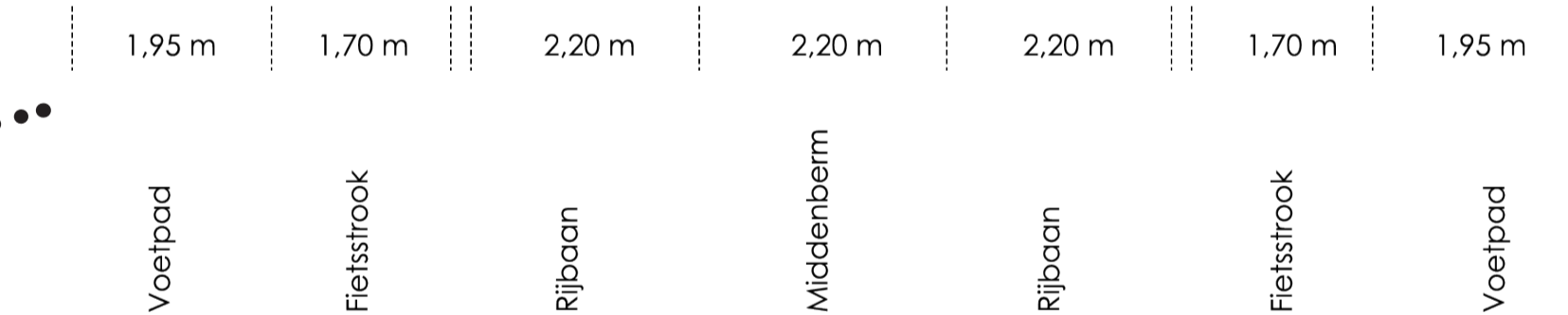
Schetsontwerp
