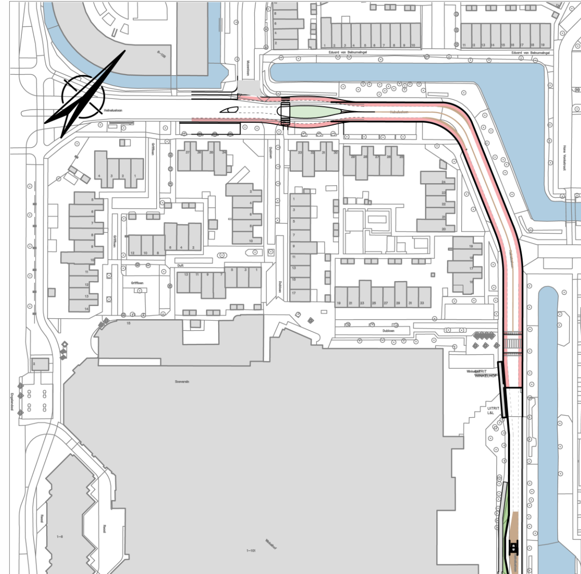
OPTIE 2 – ENTREE MET BREDE MIDDENGELIDER
