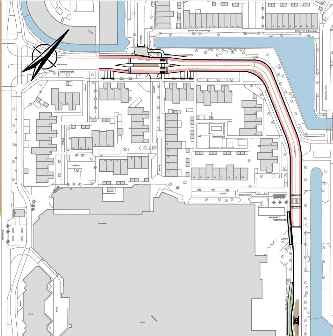
OPTIE 1 – ENTREE MET SMALLE MIDDENGELIDER
