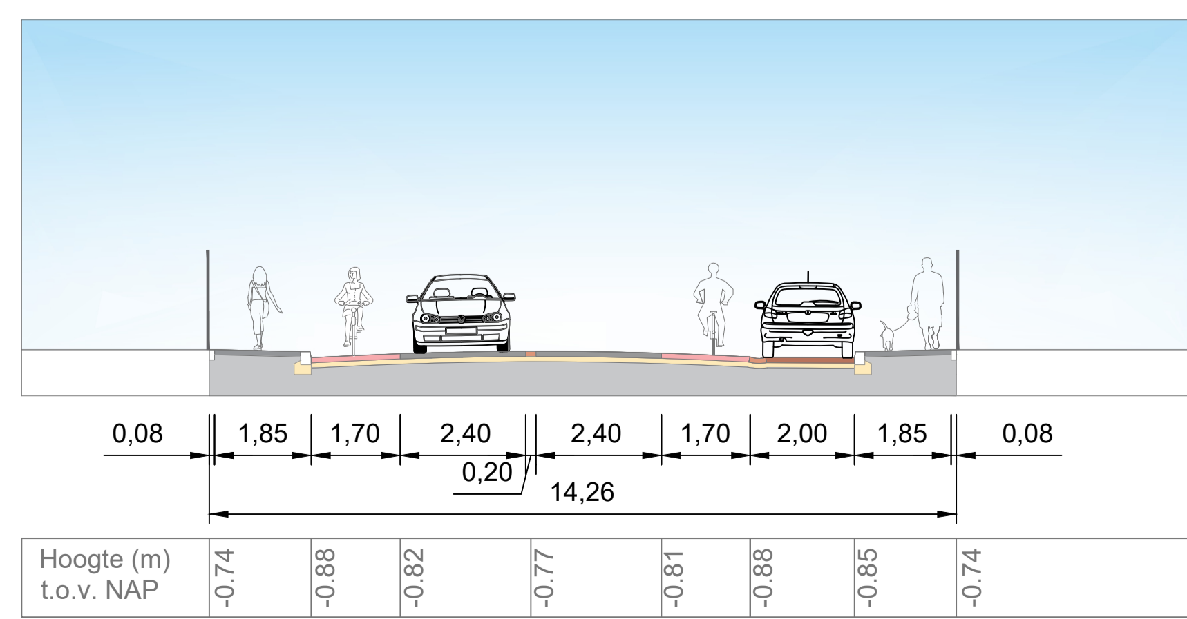
Dwarsprofiel B-B
